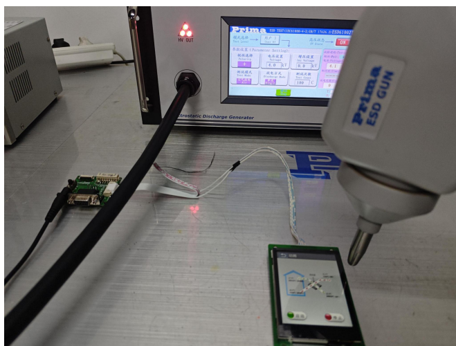
图 5-2 ESD 测试图
