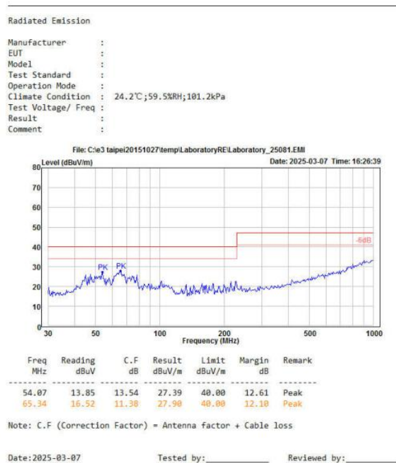
图 5-7 辐射测试垂直方向
